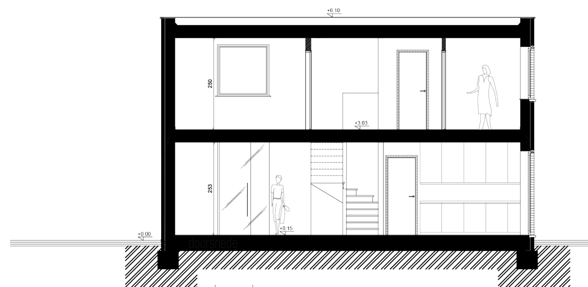
doorsnede
